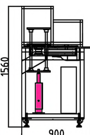
側面図
